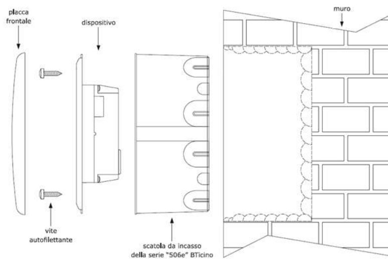
Figura 2 - Fissaggio controllo remoto V-Room
